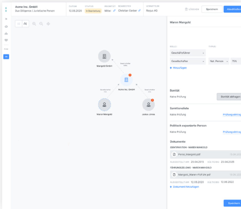
Werkzeug zur KYC- und Netzwerkanalyse auf der Grundlage von Structr und Neo4j.
